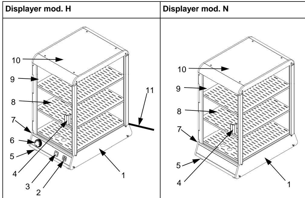
Fig.n.1 - Displayer general view
